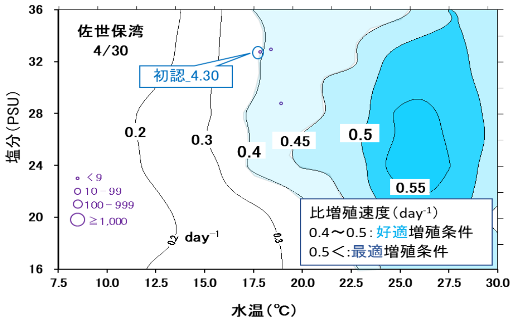
カレニアの発生量と比増殖速度( \text{day}^{-1} )に及ぼす 水温、塩分の関係
